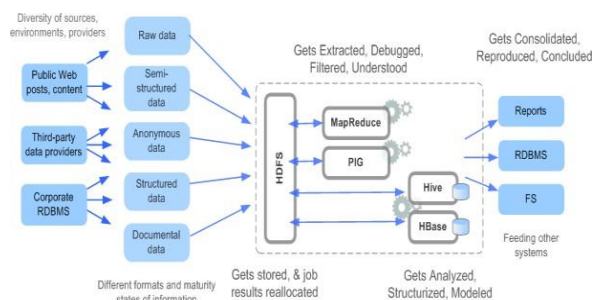
Gambar 4. Bagan Mekanisme Map Reduce Hadoop
